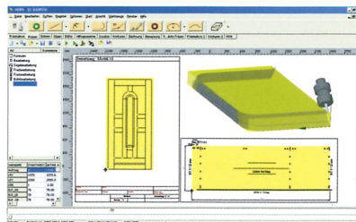
In NC-HOPS programmierte Rahmentürelemente mit 5-Achs Bearbeitung und Bewegungsplan
