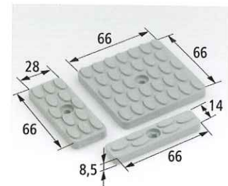
Reibplatte
