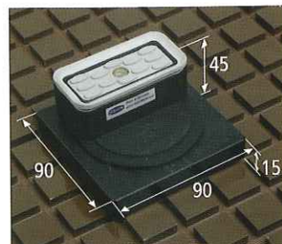
Mono-Base-R 90x90x15 mm mit Sauger-Cup 2 80x40x30 mm
