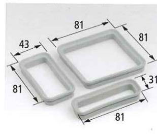
Dichtrahmen
