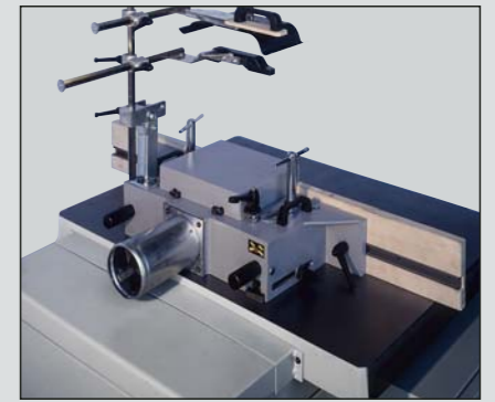
Protezione toupie registrabile Adjustable spindle protection Regulierbarer Fränschlag Protecteur toupie réglable Guia tupi regulable
