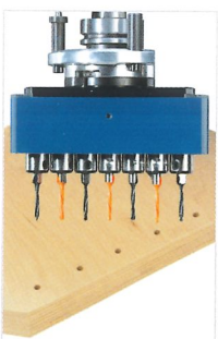
Bohren, 7 Spindeln - 25 mm Raster
