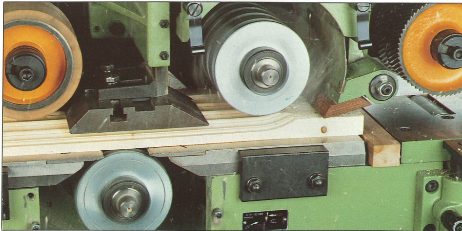
▲ Einige Gründe für den Unimat-Erfolg: Hochpräzise Arbeitsspindeln. Solide Andrücke. Solide Abführungen. Schwere Gußkonstruktion. Das ausgereifte Vorschubsystem. Das Weinig Know how.
