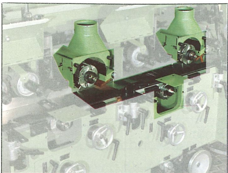
Spindelanordnung: oben – unten – oben
