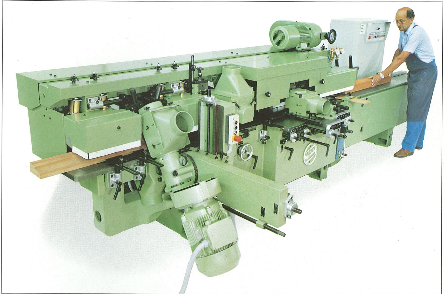
▲ Der Unimat in der Fensterfertigung: Kurze Umrüstzeiten bei kleinen Serien! Das senkt Kosten.
