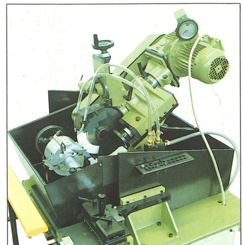
Messer-Profiliermaschine Rondamat
