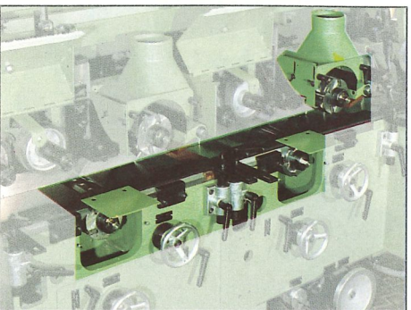
Spindelanordnung: oben – unten – unten
