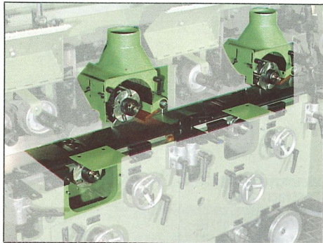
Spindelanordnung: oben – oben – unten
