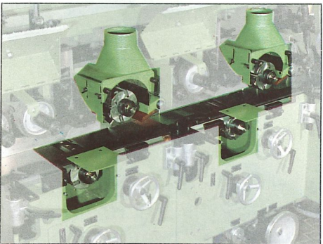
Spindelanordnung: oben – unten – oben – unten
