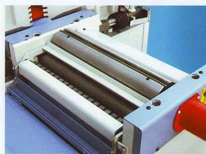
Ножов вал • Messerhobelwelle Cutter block
