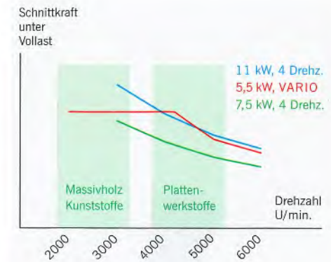
VARIO: Stufenlose Drehzahlverstellung
