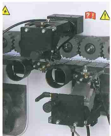
Profiliziehklängenaggregat Zum Glätten von Radien oder Fasen.
