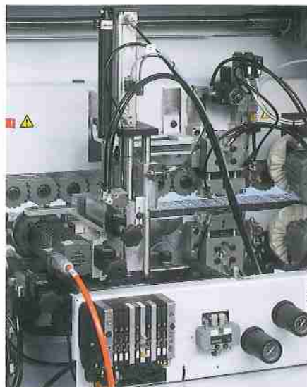
Formfräsaggregat Optimales Formfräsen ohne Einstellarbeiten durch Kopplung von DIA-Werkzeug und Tastrolle.
