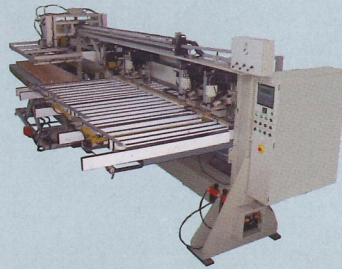
T-9/4 Taladro automático con posicionamiento de cabezales, manipulación, reenvío y apilación.
