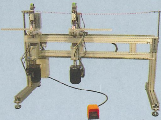
P-1 Máquina automática para taladrar los orificios de la bisagra de diámetro 35 para perfil de aluminio.
