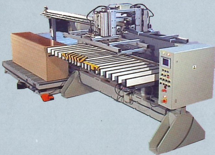
P-91 Punzonadora automática con manipulación, reenvío y apilación.
