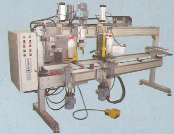
P-3 Máquina automática para cortar a 90 y 45 grados el perfil de aluminio, para realizar los agujeros del montaje del marco y hacer el agujero del tirador.
