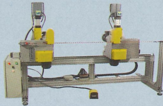
P-2 Máquina automática para taladrar y fresar los orificios de la bisagra oculta para perfil de aluminio.
