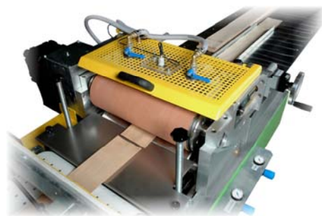
Walzenauftragsystem für Weißleim
