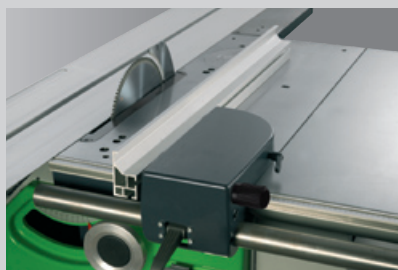
Parallelanschlag
