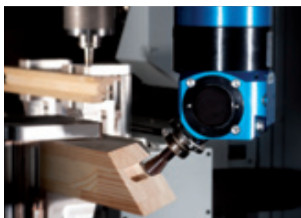
Exakte Schifterschnitte und Eckverbindungen – passgenau auf Anrieb.
