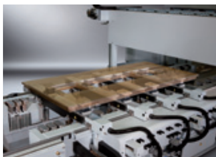
Die universellen Spannsysteme können simultan eingesetzt werden – z. B. für die Haustüren oder Rundbogenfertigung.
