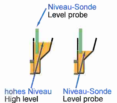
Auftragseinheit glue application unit
