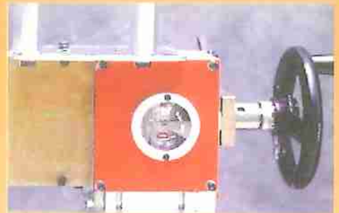
Particolare di lettura su nastro millimetrato ingrandito. Detail of reading from enlarged measuring rod. Détail de lecture sur bande millimétrée agrandie.
