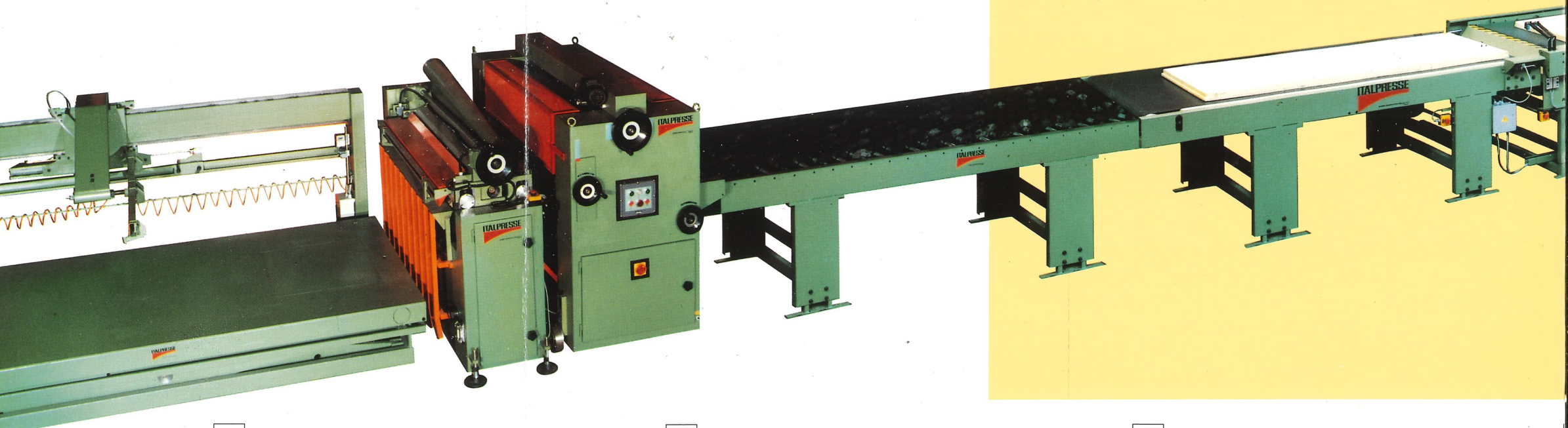
1 POSIZIONAMENTO SU VANO POSITIONIERUNG AUF DER ETAGE
