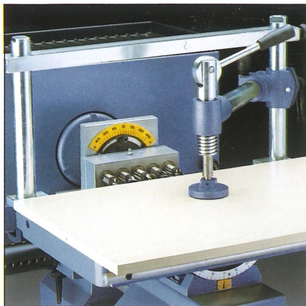
Mehrspindelbohrkopf
