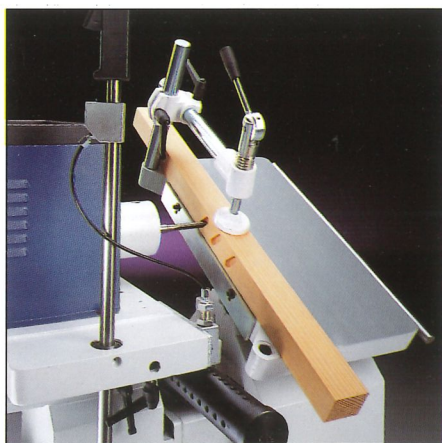
Schrägstellbarer Tisch bis 45°
