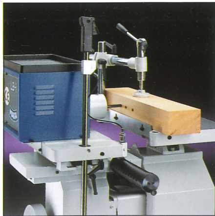
Dübellochbohrereinrichtung mit Schnellverstellung
