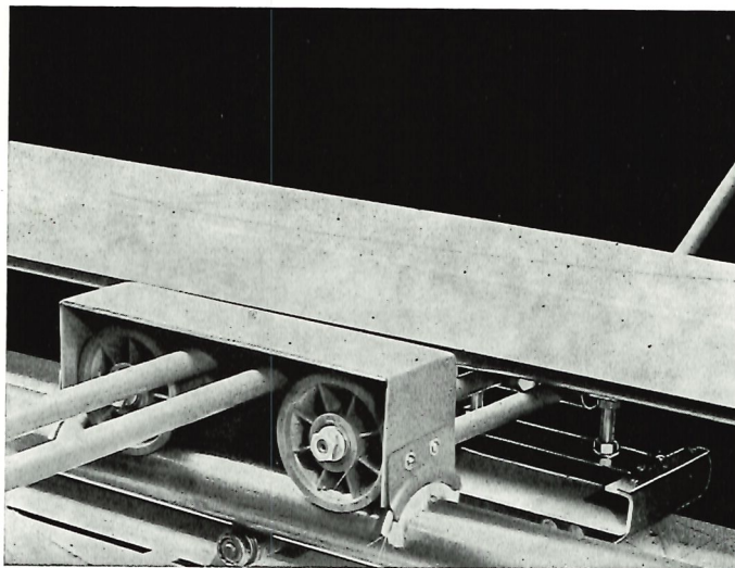
Schleifschuhträger
