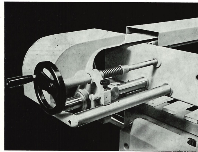
Schleifbeltspannvorrichtung
