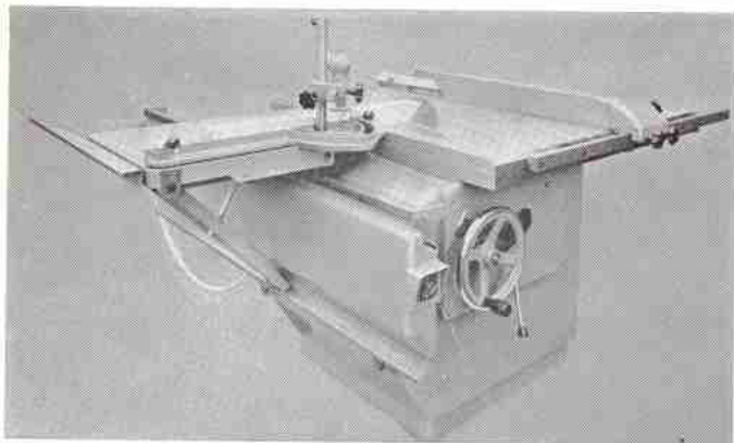
Schwere schwenkbare Hochleistungs- Tischkreissäge Typ SKS-45
