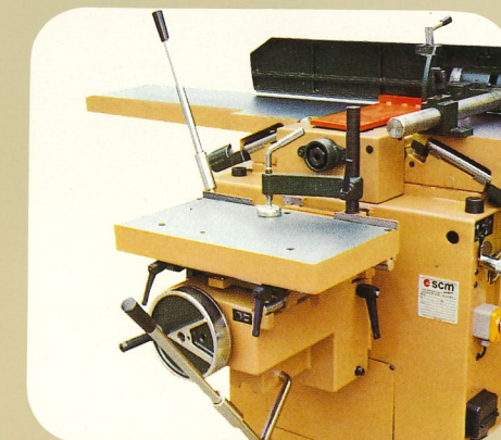
Mortaiseuse. Langlochbohrereinrichtung.
