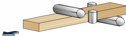
Maschinenausführung mit 4 Spindeln und mit 10 mm Profiliertiefe auf den Vertikalspindeln.
