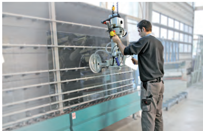
Vakuum-Hebegerät VacuMaster Window bei der vertikalen Handhabung einer Glasscheibe
