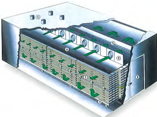
蒸汽式烘房
