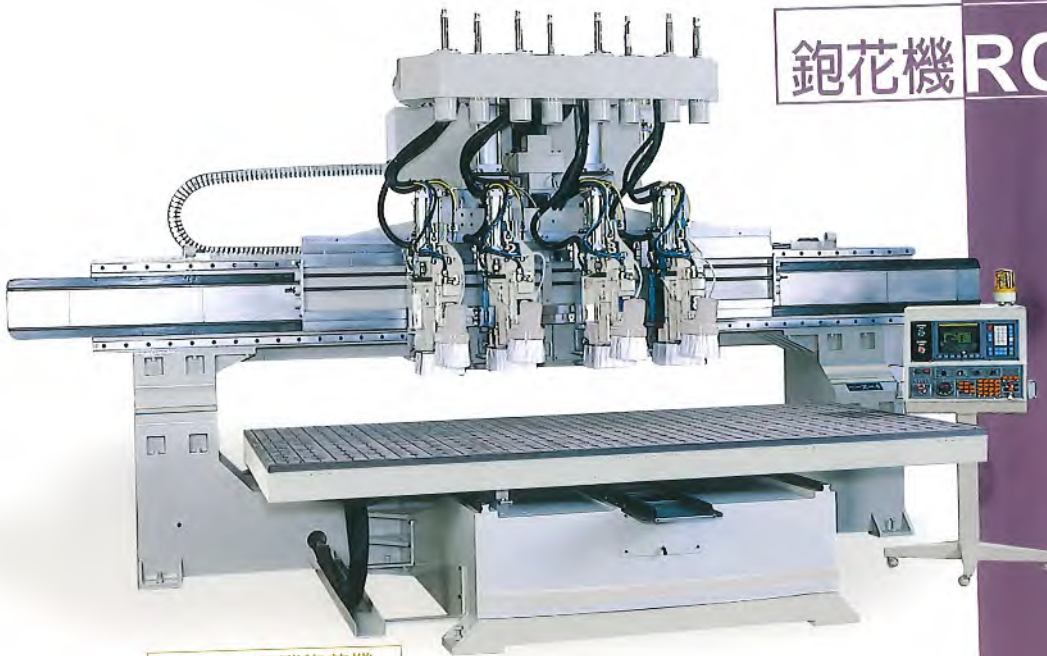
CNC電腦鉋花機 CNC Router
