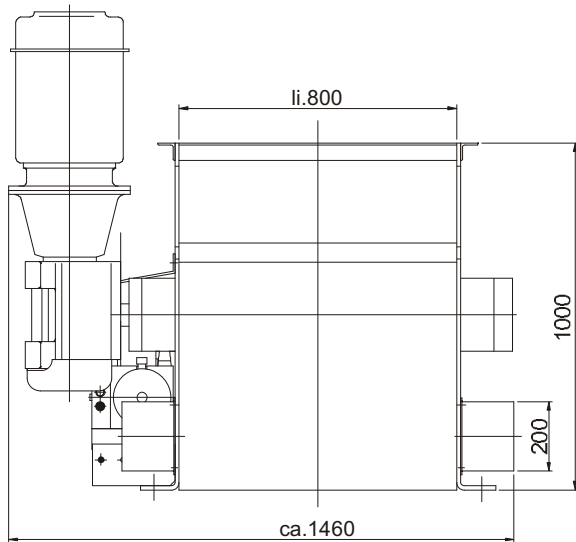
Frontansicht · front view · vue de face
