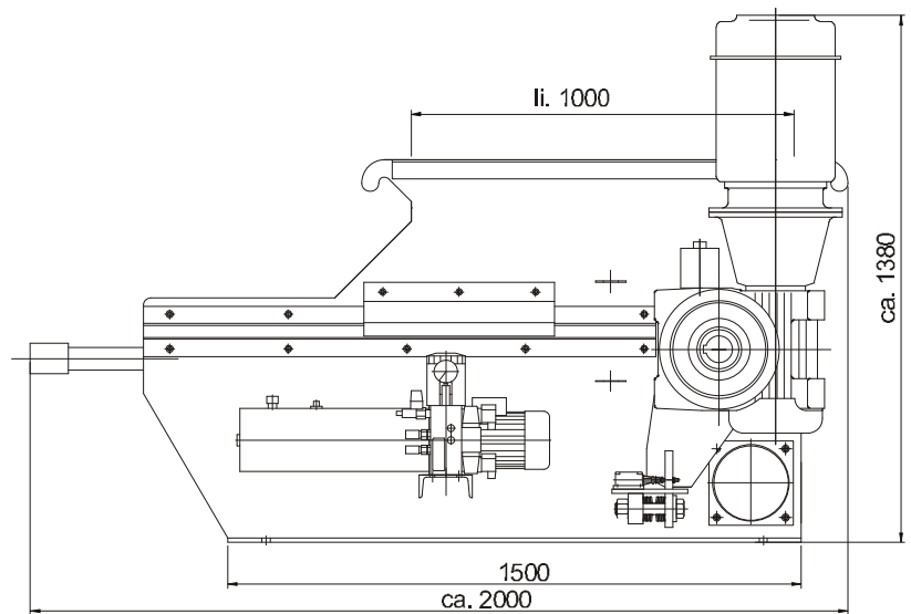
Seitenansicht · side view · vue de coté
