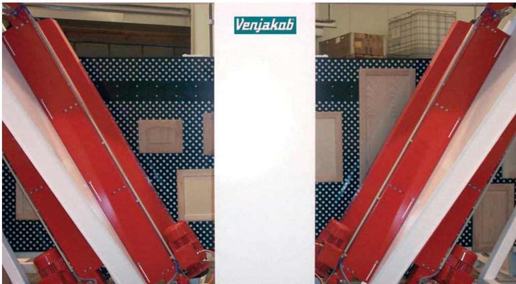
Beizevertreibermaschine für vertikal geförderte Werkstücke mit Vakuumtransportband.
