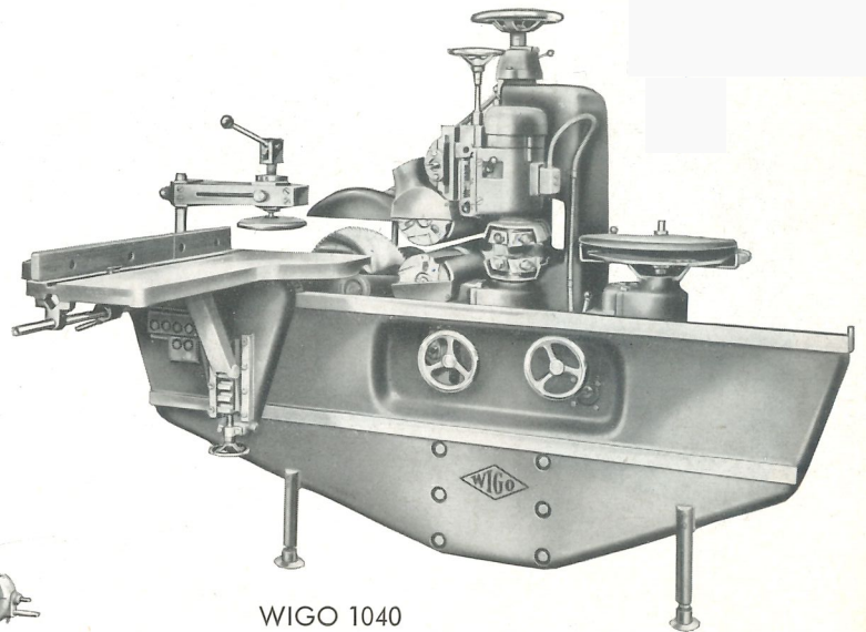
Zapfenschneid- und Schlitzmaschine
