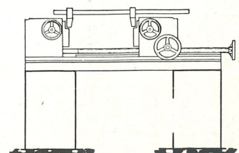
Doppel-Ablängsäge für Kleinformat
