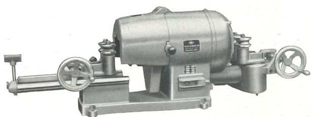
Halbautomatische Rundstabhobelmaschine WIGO 1060
