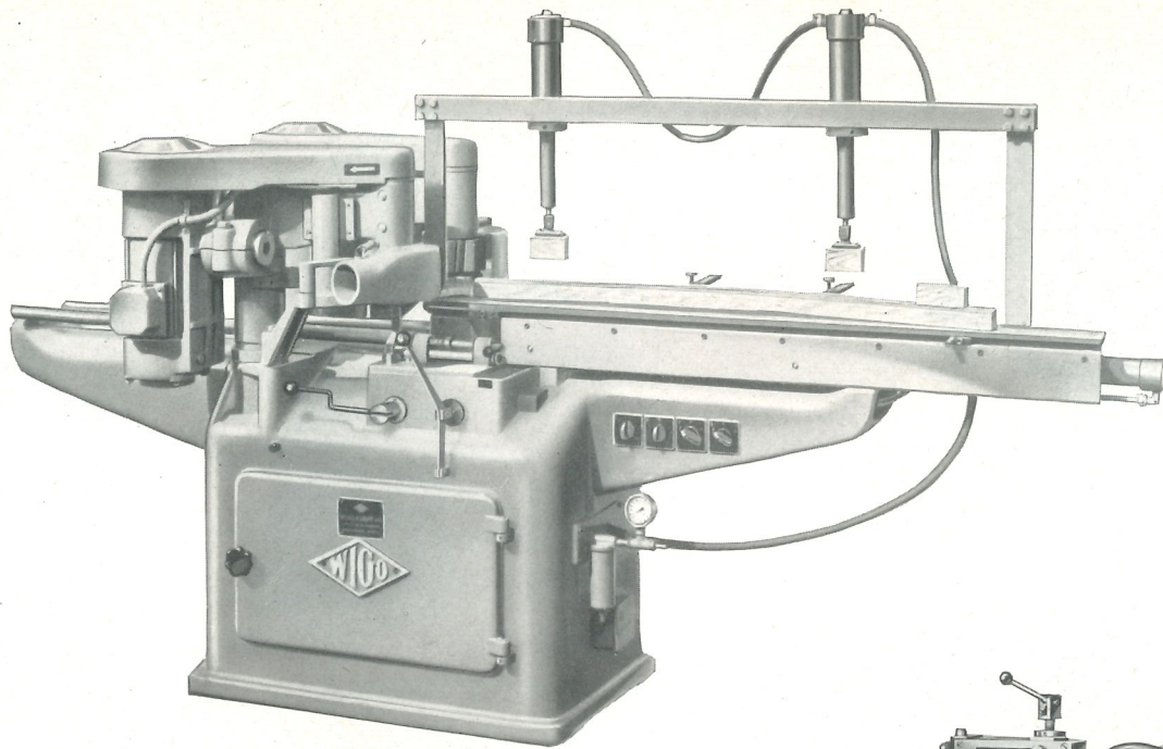
Autom. hydr. Doppel-Kopierfräsmaschine WIGO 1075
