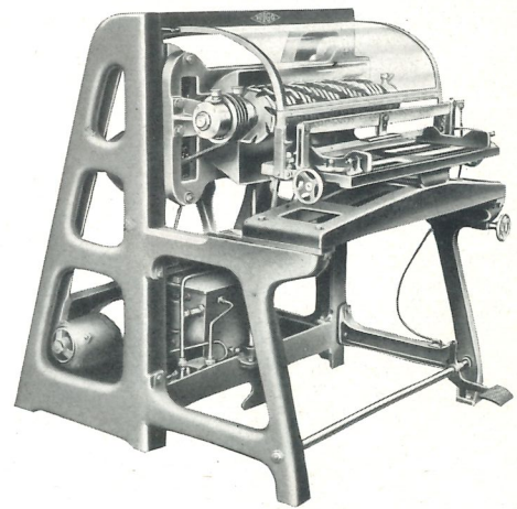
Hochleistungs-Zinkenfräsmaschine WIGO 1016
