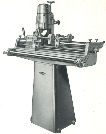
Hochleistungs-Zinkenfräsmaschine WIGO 1016
