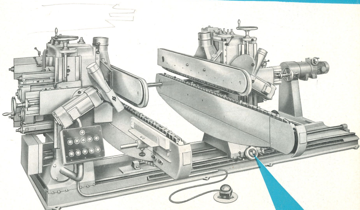
Doppelendprofiler WIGO 1031 A/B
