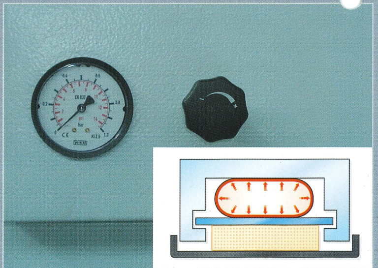
Einfache Regulierung des Schleifdrucks im Luftkissen-Schleifschuh
