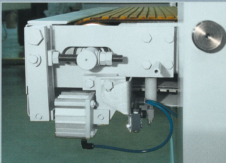
Automatische Gurtsteuerung
