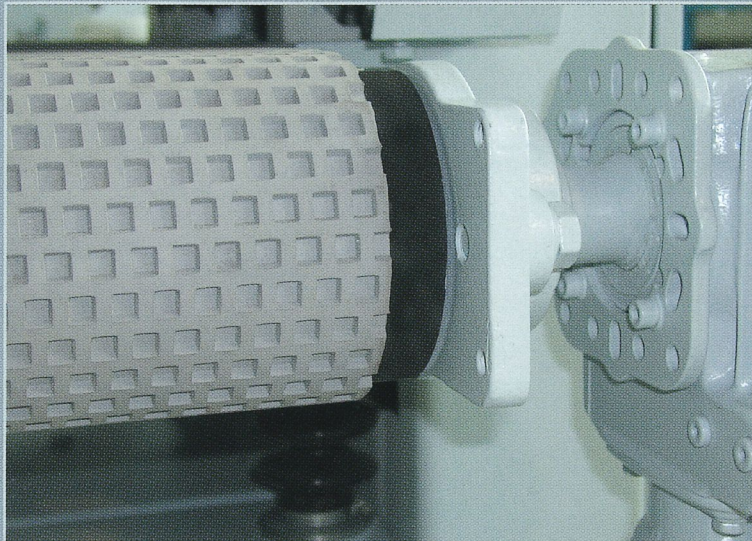
Gummierte Gurtantriebstrommel
