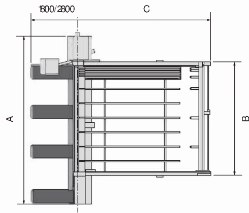
AXO300 / AXO400
