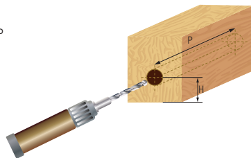
Perforación en cantos
