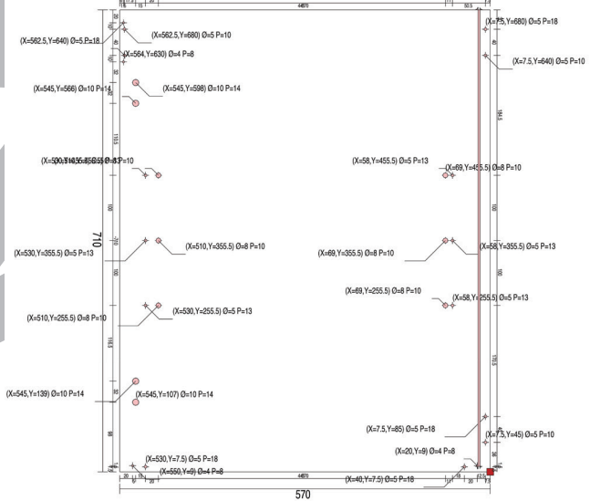
Ranuras con disco
