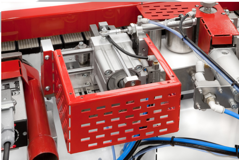
Retestador con cuchilla (MYKRO PLUS)
