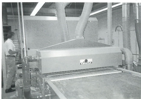
Nach der Kreuzschliffmaschine: Abblasen mit der ERNST AB2
