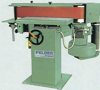
Edge Sanding Machine F 650
