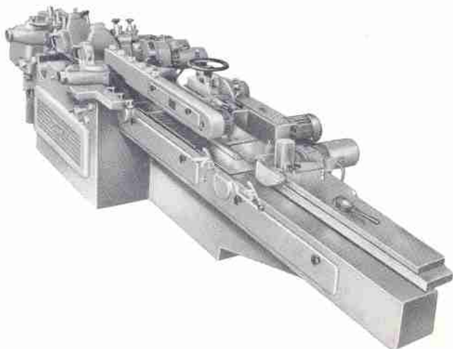
Vierseiten-Kehlmaschine mit Abricht- und Fügevorrichtung, Modell GS-9-180 · 9 Arbeitswellen · Arbeitsbreite 200 mm
