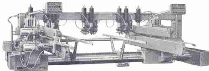
Schwere zweiseitige Zapfenschneid- und Schlitzmaschine Typ LSQTDE · Vorrichtungen zum Bohren · 6, 8, 10 und 12 Arbeitsspindeln
