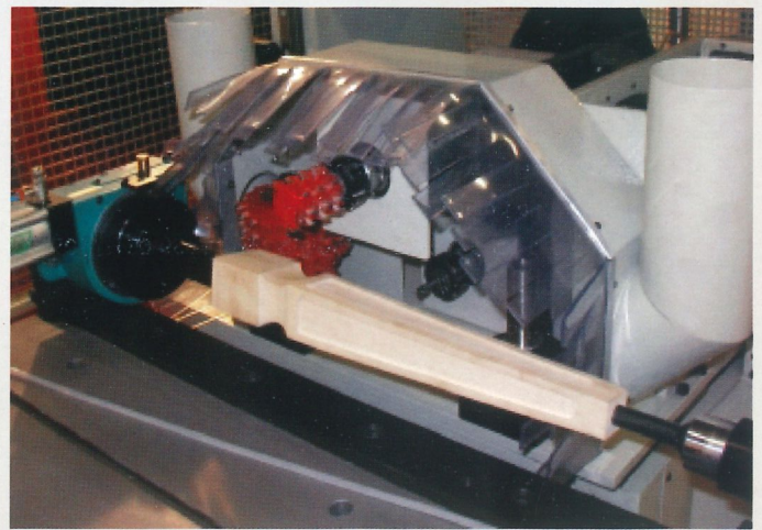
Divisore a 4-8 posizioni Divisor at 4-8 positions Diviseur à 4-8 positions Drehvorrichtung mit 4-8 Stellungen Torno a 4-8 posiciones
