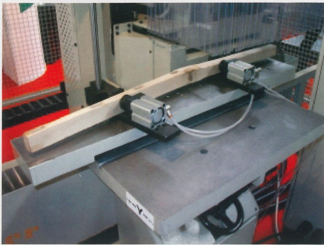
Gira-pezzo da 0° a 90° 0-90° rotating device Dispositif tourne-pièce de 0° jusqu' à 90° Klapptische 0-90° Mecanismo vuelta-pieza de 0 a 90°
