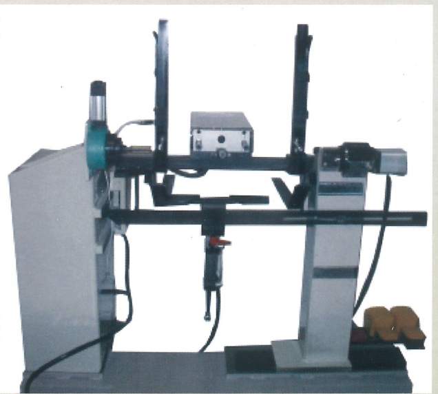
Caricatore automatico completo di divisore Automatic hopper-feed complete with divisor Chargeur complet de diviseur Ladungsmagazin mit Drehvorrichtung Cargador automatico completo de torno
