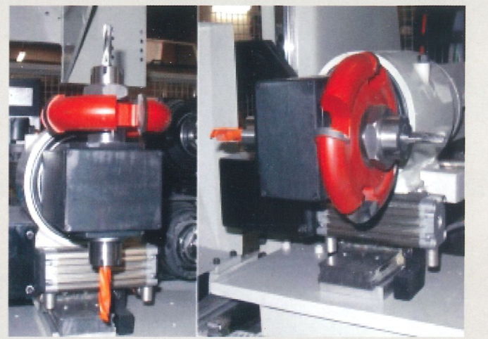
Unita speciale con rotazione 0-90° e a doppia uscita Special unit rotating 0-90° with 2 spindles Unité spéciale avec rotation 0-90° à 2 sorties Spezielles Aggregat, schwenkbar um 0-90°, mit 2 Austritten Unidad especial con rotación 0-90° y a double salida
