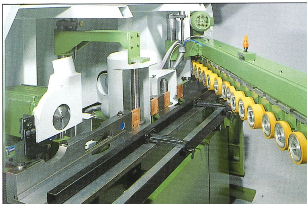
- kettenloser Vorschub - Gleichlauf-Eintauchaggregat - Fräsaggregat. Gegenlauf, für 3 Werkzeuge - Nutfräsaggregat - chainless feed - clockwise diving automatic - profile spindle counter-clockwise for 3 sets of tools - groove cutter
