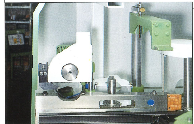
- Glasleistensägeaggregat - automatisch getaktetes Stützlineal für Glasleistenaustrennung - glass bead recovery - automatically cycled support for glass bead removal
