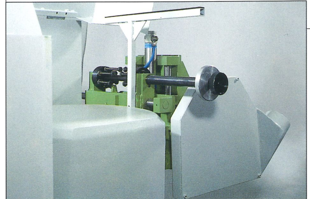
- Ablängsäge automatisch von oben eintauchend - pneum. Horizontalverstellung - Revolveranschlag für 12 Positionen - sizing saw autom. diving from above - pneum. horizontal adjustment - Revolving unit for 12 positions
