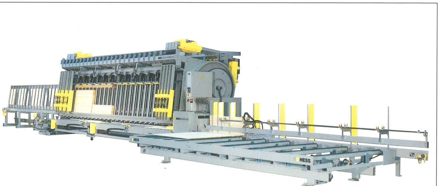
VERLEIM-SYSTEM 2000 Vorsortierstation, Beileimlinie, Verleimrotor, Übergabestation
