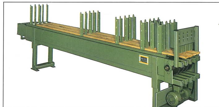
1-4teilige Magazinbänder
