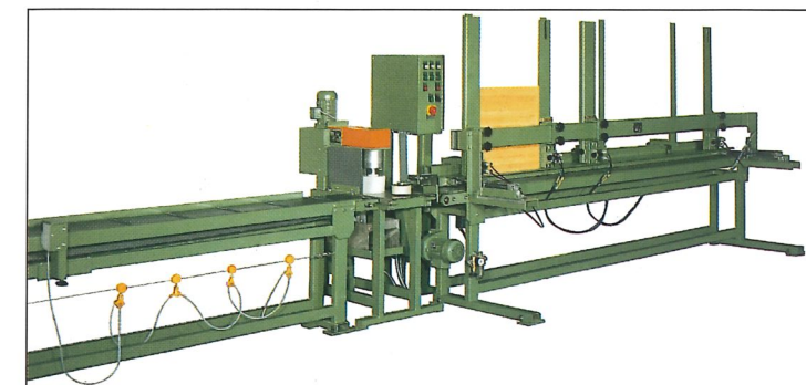
Magazinband, Beilemstation, Stollenförderband
