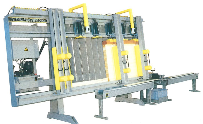
. . . oder mit Beleimlinie (hier Einfachversion)
