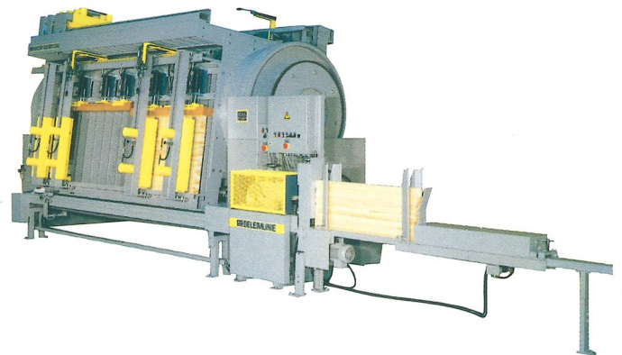
. . . als Verleimrotor . . .
