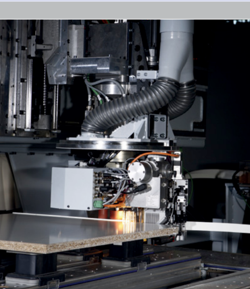
Placage laserTec pour des pièces de forme au jointage optimal
