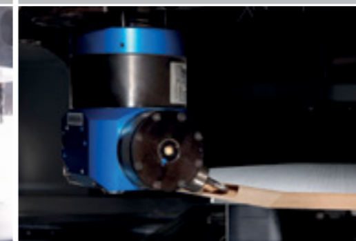
Usinage quelque soit l'angle avec l'agrégat FLEX5+
