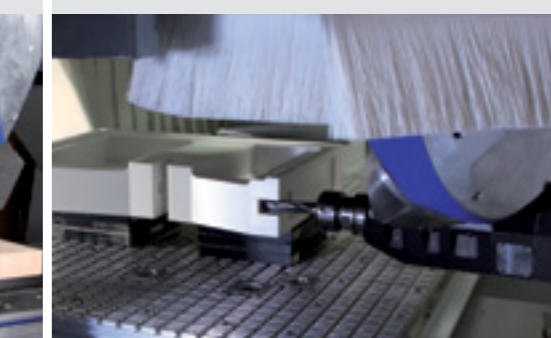
Fraisage de composants machine
