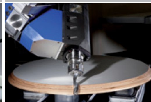
Fraisage de chanfrein sur un dessus de table
