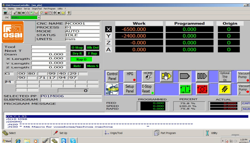
Bild 12. OSAI Steuerung
