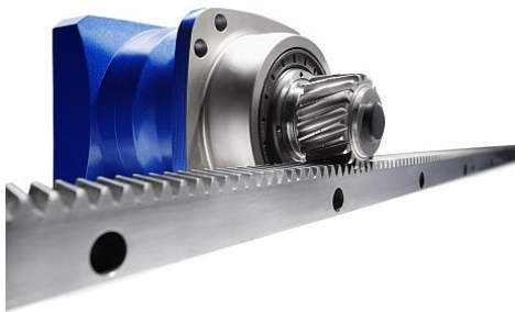
Bild 3. Zahnstangen— RitzelantriebOb mit SHIMPO Getriebe Antrieb
