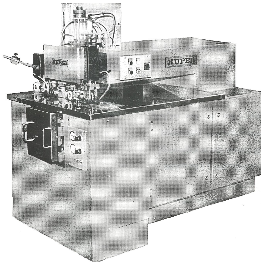
Furnier- Zusammensetzmaschine FW/L 920
