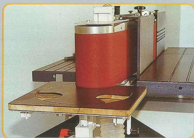
Doppelseitige Kantenschleifmaschine Double ended edge sanding machine
