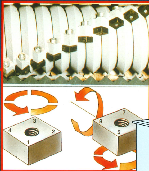
Der Spiralrotor (ziehender Schnitt = geringer Kraftaufwand) ist mit Spezial-Wendebrechplatten bestückt.
