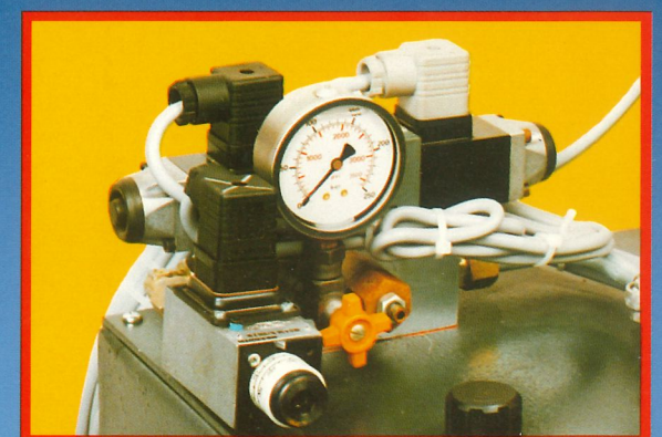
Das Hydraulikaggregat wird wahlweise auf dem Maschinenkörper montiert oder verdeckt eingebaut.
