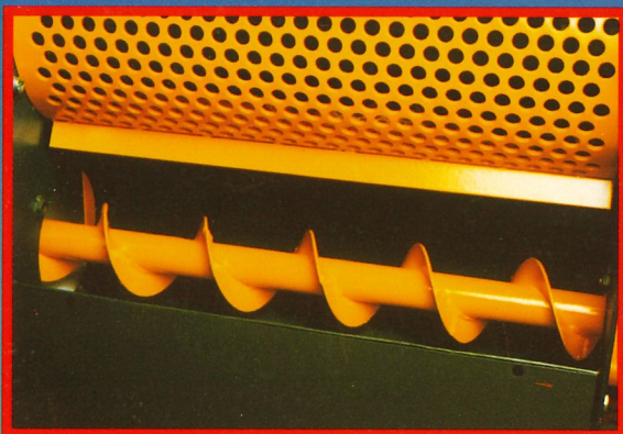
Auf Wunsch kann eine Transportschnecke eingebaut werden (nachrüstbar).
