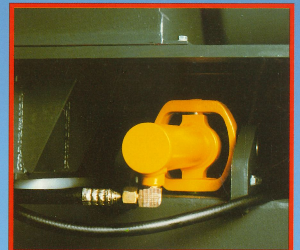
Die kardanische Aufhängung des Hydraulikzylinders federt Querkräfte ab.
