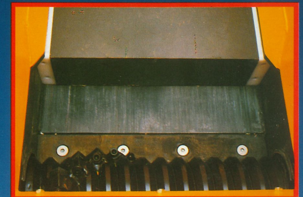
Hydraulisch gesteuertes Vorschubaggregat mit innenliegenden Führungen aus Spezialkunststoff.
