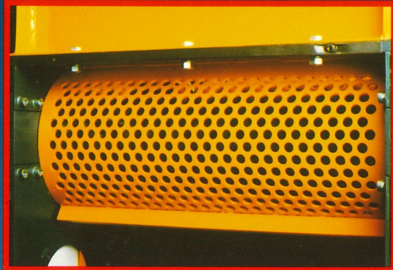
Das austauschbare Spezialsieb gewährleistet einen homogenen Span.
