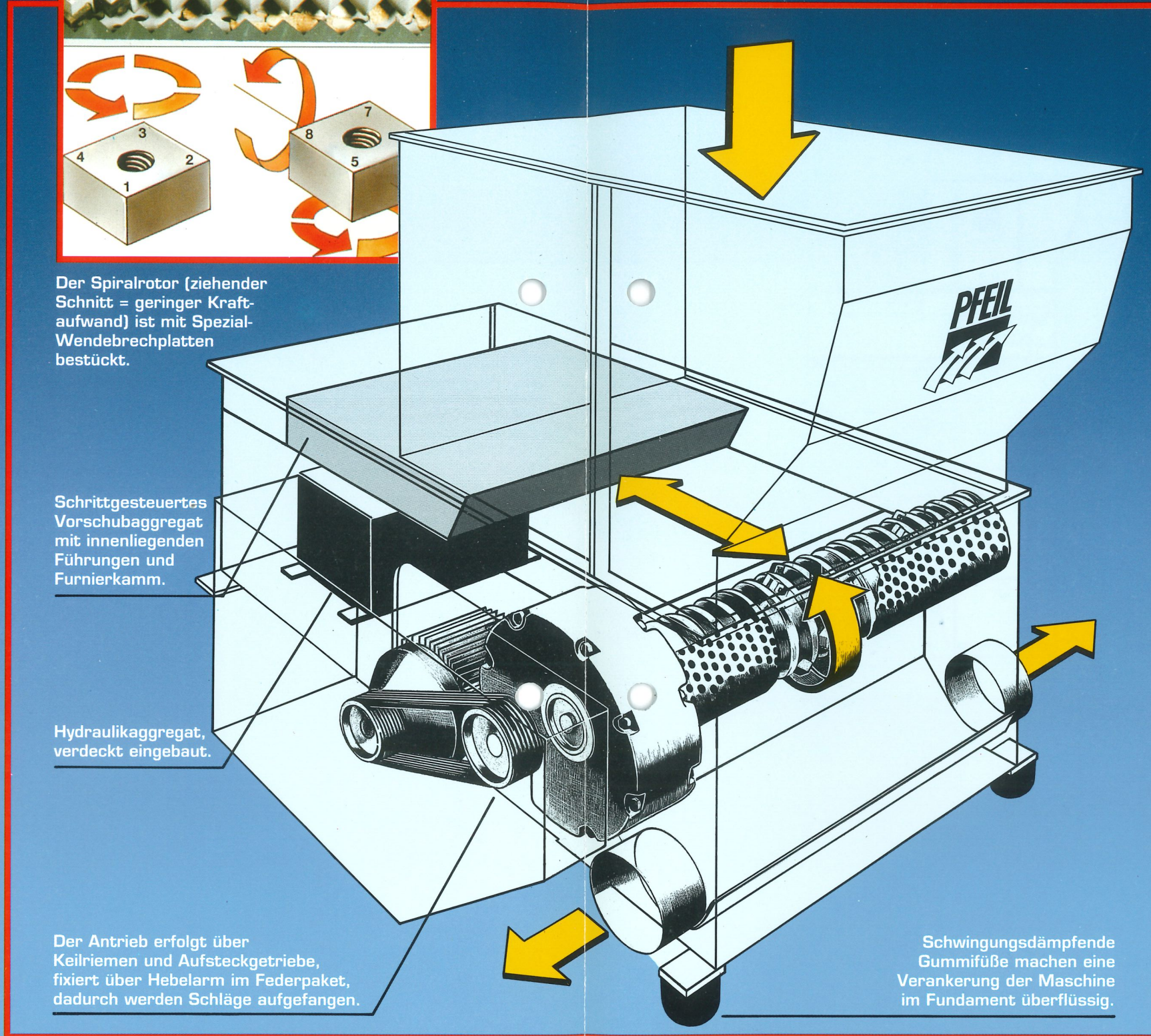
Schematische Darstellung einer Pfeil-Zerkleinerungsmaschine.
