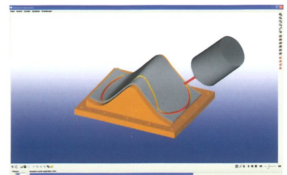
In AlphaCAM programmiertes 5-achsiges Besäumen mit der Werkzeugflanke
