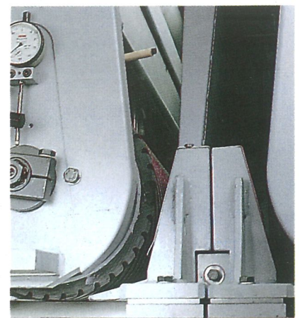
Schwere Gußdruckbalken garantieren genaue Werkstückführung und erlauben die Bearbeitung von kurzen Teilen
