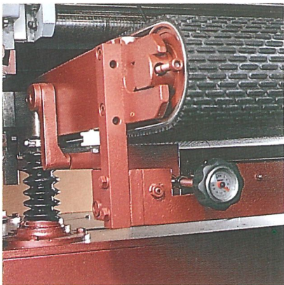
Tischfederung mit Feineinstellung
