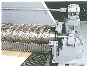
Hobelaggregat (abgebildet ohne Abdeckung)
