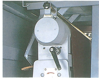
Bandabbläsung
