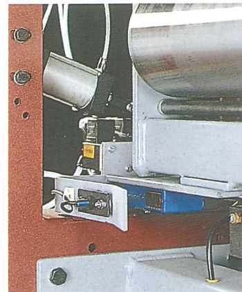
Electronische Schleifbandoszillation
