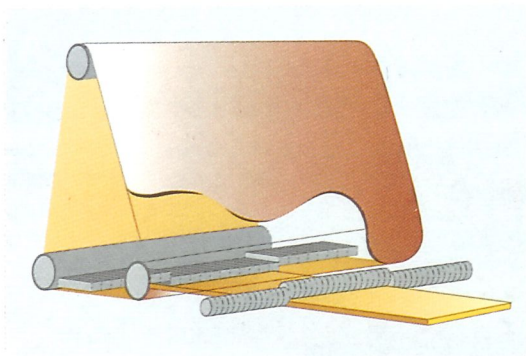
Segmentschleifschuh (schematisch)
