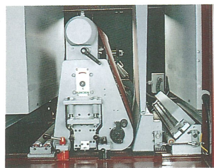
1-Band-Kombi-Maschine mit Segmentschleifschuh
