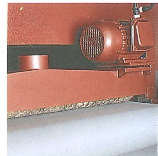
Werkstückreinigungsbürste (auch Transportbandreinigungs- bürste verfügbar)
