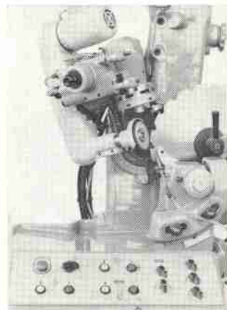
Feinstschleifautomat ASHK-MAXI- MAT B: Automatischer Rückenschliff eines wechselseitig schräg geschlif- fenen Hartmetallsägeblattes
