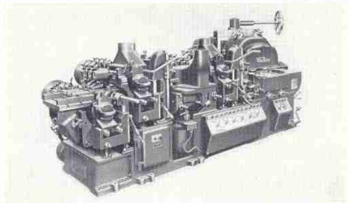
Hobel- und Kehlmaschine Typ FDF · Arbeitsbereich 305 \times 152 mm
