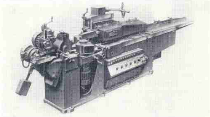
Langtischkehlmaschine Typ FZ · Arbeitsbereich 157x157 mm
