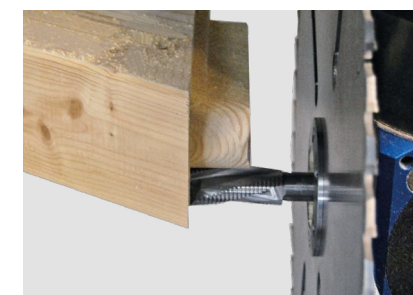
Zapfenverbindung
