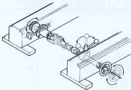
Bloccaggio meccanico Mechanical locking Serrage mecanique
