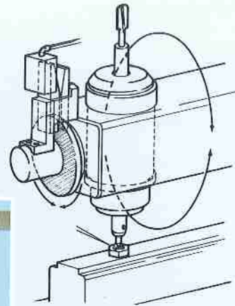
Motore reversibile e freno a disco a bloccaggio pneumatico regolabile Reversible motor and presetting disc brake for pneumatic locking Moteur reversible et frein à disque reglable à serrage pneumatique
