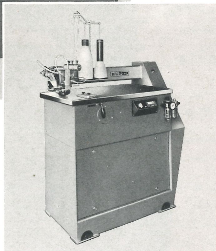
EMZ/1, Endverklebemaschine EMZ/1, Veneer End Splicer EMZ/1, Jointeuse à border les placages EMZ/1, máquina repasadora de chapas por los extremos ▶
