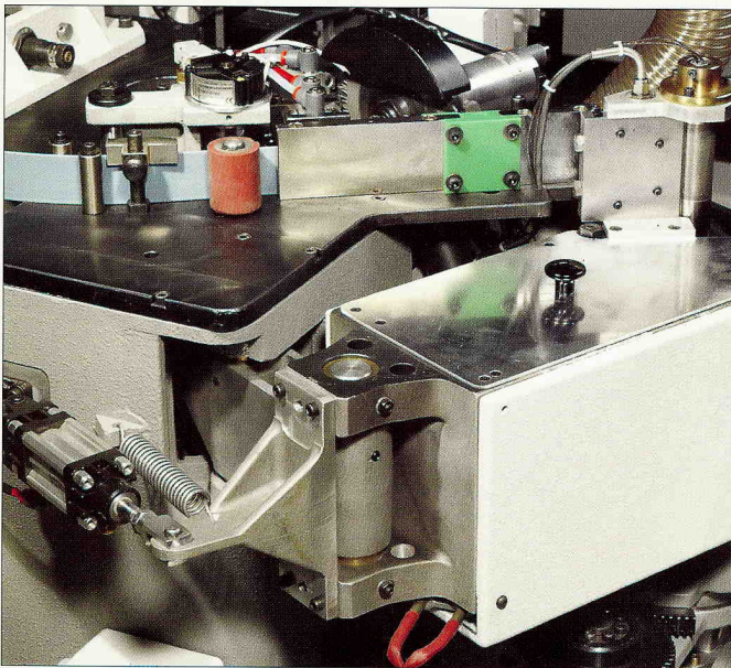
Edge-banding unit. Kantenanleimaggregat.
