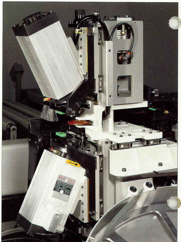
Double edge-trimming unit. Doppel-Vorfräs/Bündigfräsaggregat.
