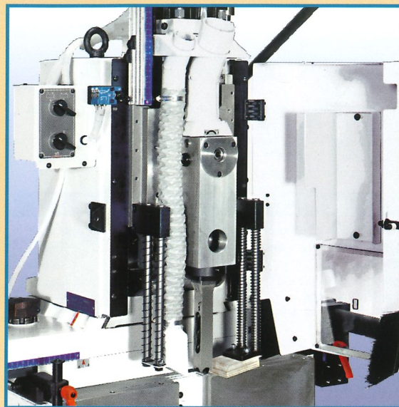
Particolare dell'unità porta-bedano. Detail de l'unité porte-bedano. View of chisel-holder unit. Detailansicht des Lochbeitelaggregates.
